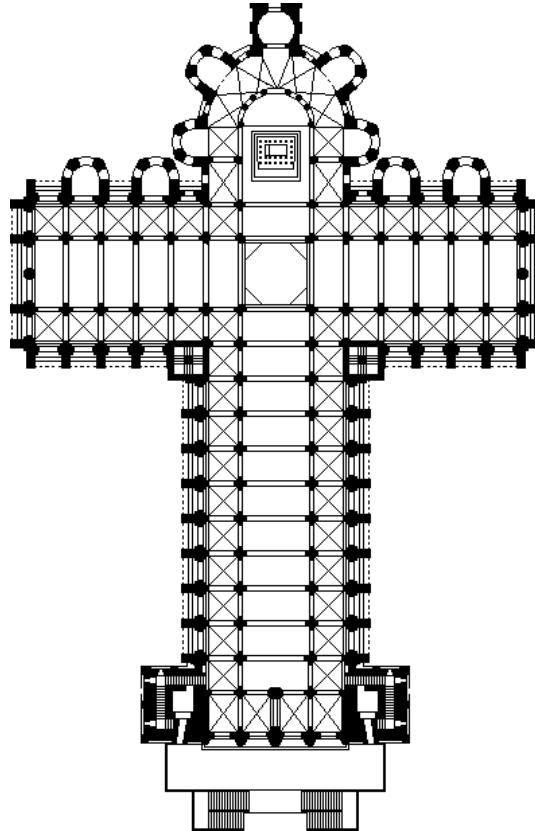
Fig. 1: Planta de la Iglesia de Santiago de Compostela 1
